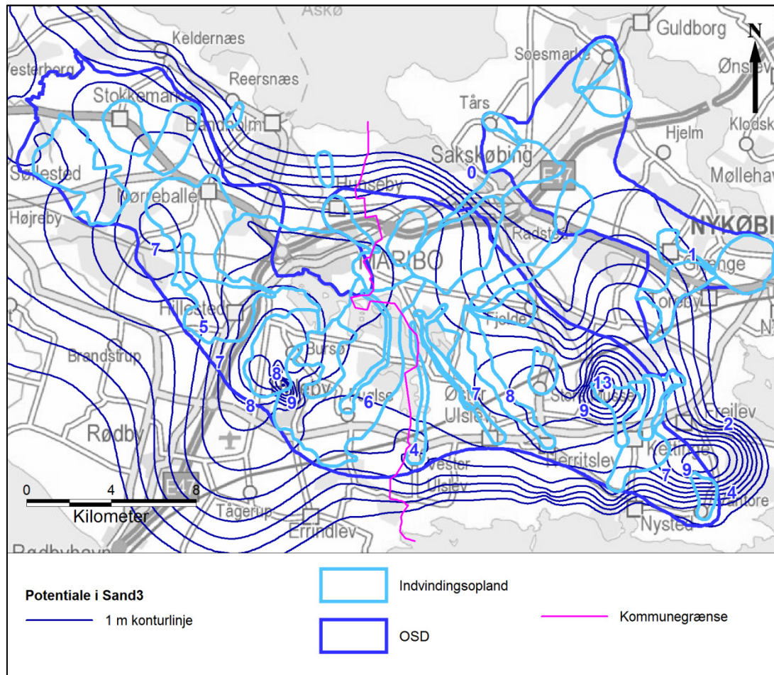
Figur 7 Potentialet i Sand 3 magasinet baseret på målte potentialer fra synkronpejlerunde i 2012. Grundvandet strømmer vinkelret på konturlinjerner, fra områder med højt potentiale mod områder med lavere potentiale.
