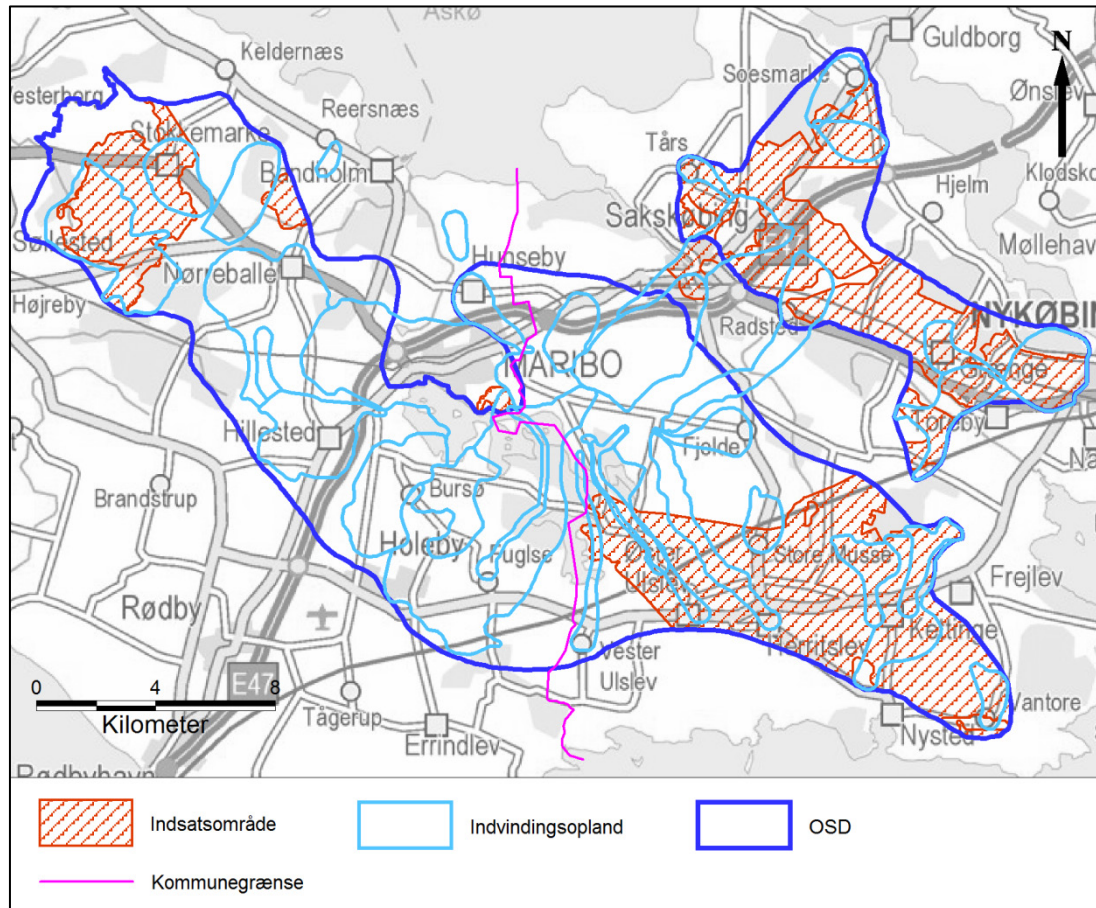
Figur 11 Indsatsområder (IO) med hensyn til nitrat jf. Redegørelsen for Lolland. Bemærk, at der efterfølgende er blevet foretaget en genvurdering af IO i indvindingsoplandene til Reersnæs Vandværk, Rørmark Skov Kildeplads og Søllested Vandværk, se. afsnit 5 og Figur 12.
